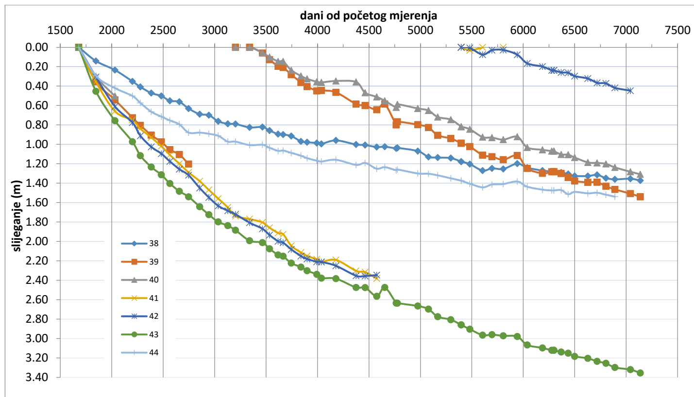
Slika 7. Prikaz konsolidacije repera broj 38, 39, 40, 41, 42, 43, 44 (profil 12). Horizontalna os prikazuje vrijeme u danima, a vertikalna os prikazuje slijeganje u metrima. Vrijeme je prikazano u linearnom mjerilu. Početni datum mjerenja slijeganja je 30.06.2011. Početni datum mjerenja slijeganja repera br. 42 je 03.09.2021.
